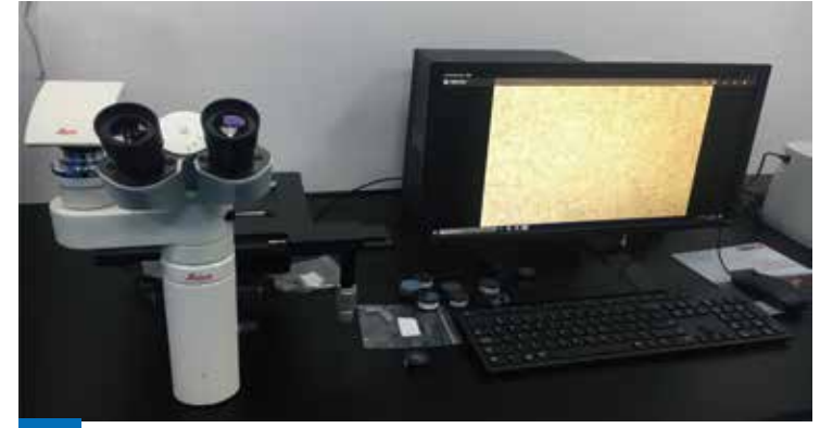
德国莱卡Leica DM ILM倒置金相显微镜 强大的图像获取和分析软件可以支持客户对金相样品的特殊观察。 Germany Leica DM ILM Inverted Microscope
